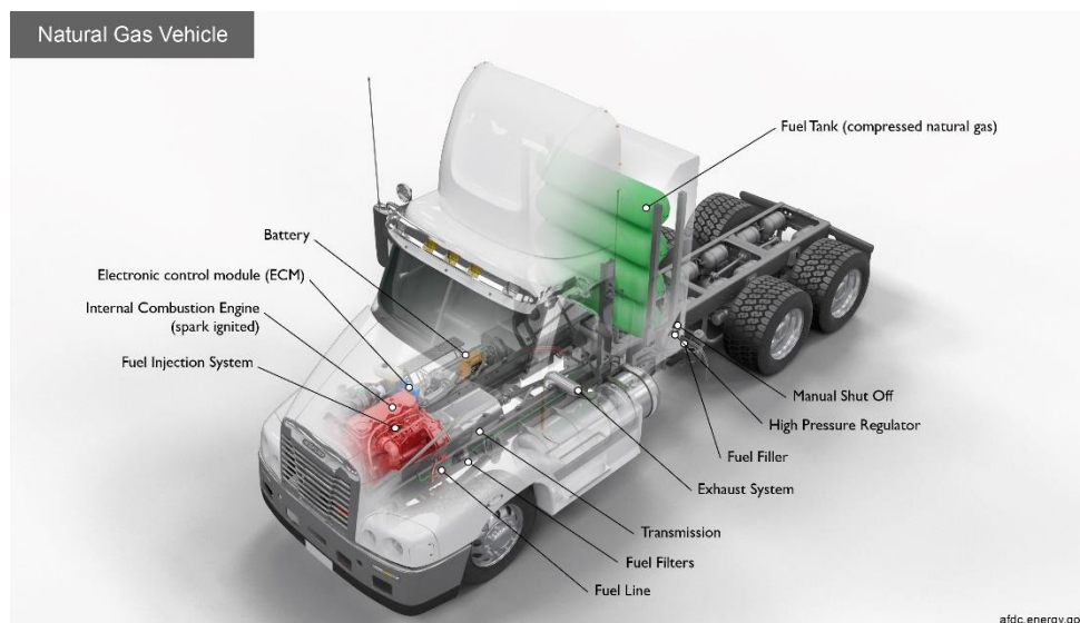
Abbildung 5 Gasfahrzeug ( afdc.energy.gov )
